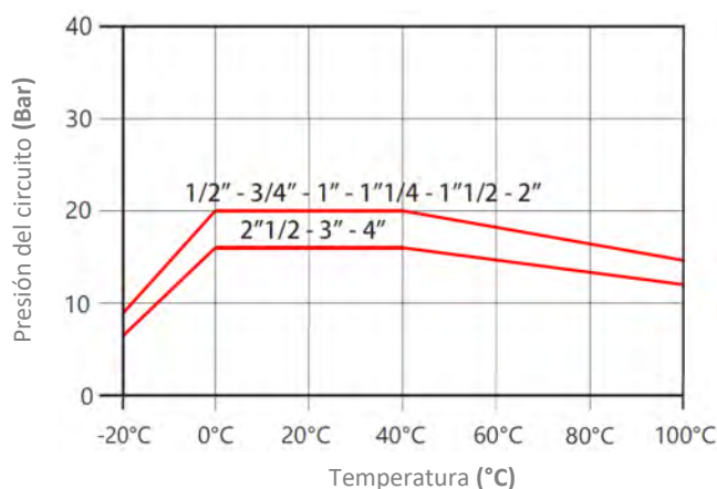
Diagrama 2: Temperatura/presión
